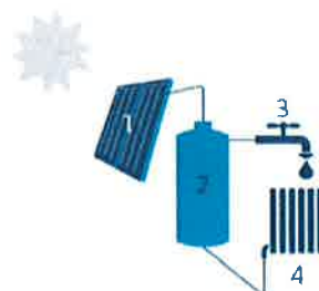
1. Zonnecollector | 2. Opslagvat zonneboiler | 3. Sanitair warm water | 4. Afgifte-element voor ruimteverwarming (opioneel)
